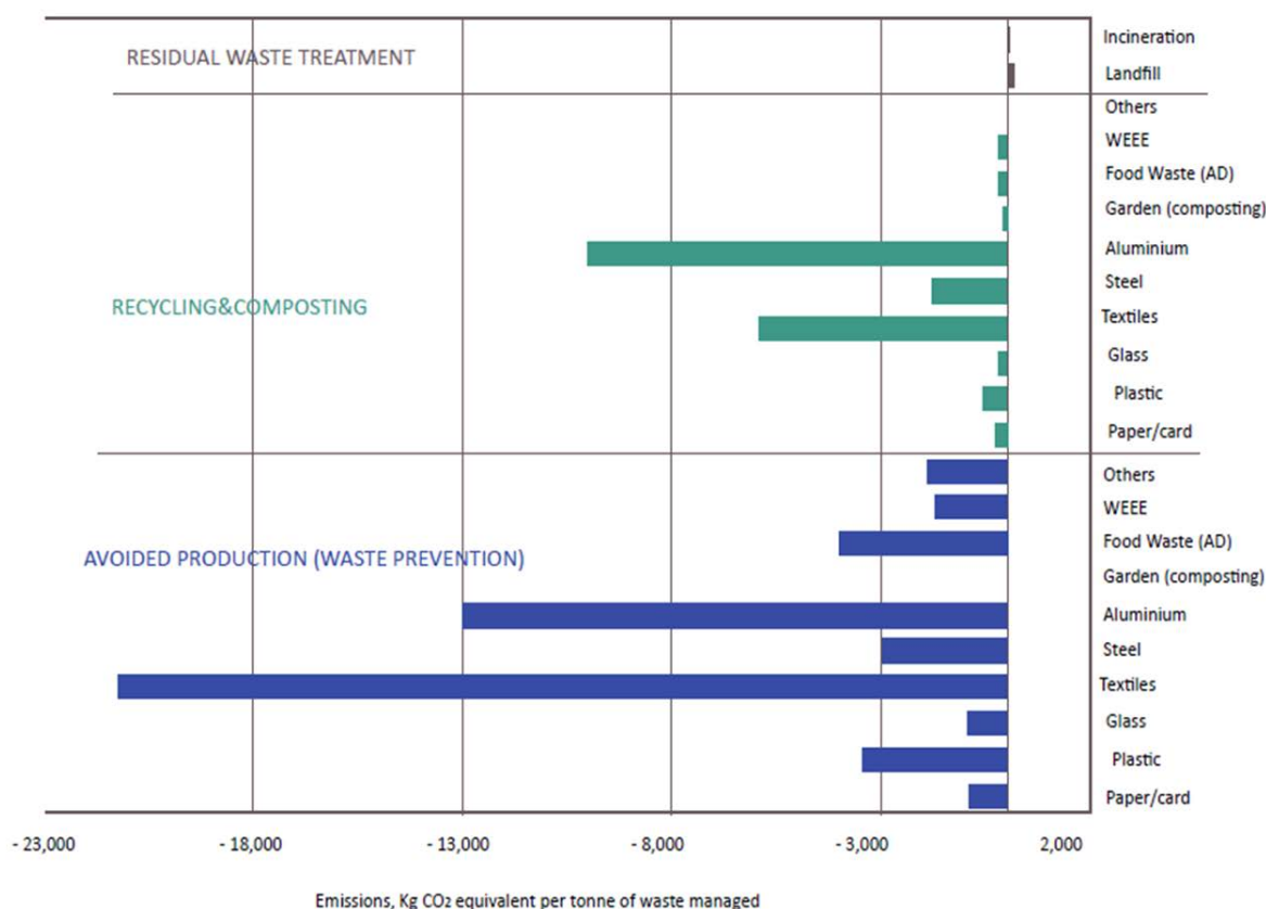
شکل ۲۱ - مقایسه میزان انتشار \text{CO}_2\text{-eq} (کیلوگرم) در اجرای هر یک از فرآورده‌های اجتناب از تولید پسماند، بازیافت و دفع بر هر تن از انواع پسماندها
